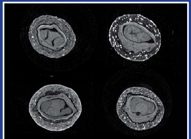
Observation de la qualité d'application de l'enrobage par radiographie (source : Fr. Strube)
